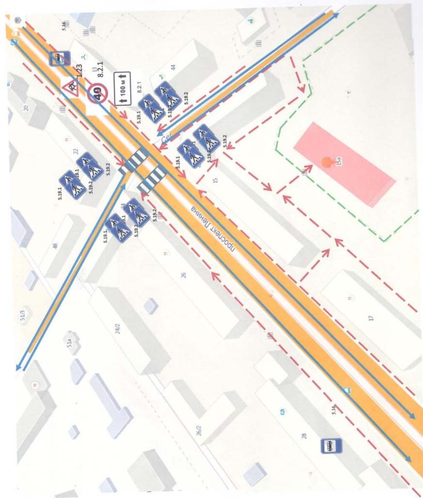
2. Схема организации дорожного движения в непосредственной близости от образовательного учреждения с размещением соответствующих технических средств, маршруты движения детей и расположения парковочных мест
